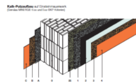
RÖFIX Aussenputz Detailzeichnungen Monolithisches Einsteinauerwerk
