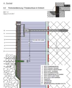
RÖFIX Aussenputz Detailzeichnungen Monolithisches Einsteinauerwerk
