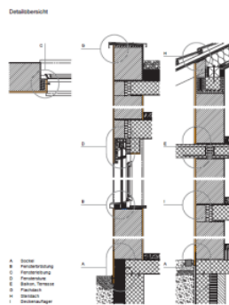
RÖFIX Aussenputz Detailzeichnungen Monolithisches Einsteinauerwerk
